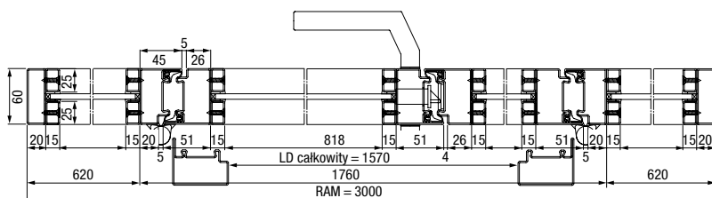
2-skrzydłowe stalowe drzwi loftowe z naświetlami bocznymi, przekrój poziomy
